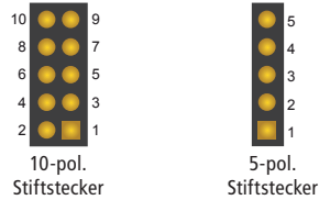
Abb. 10: Stiftstecker (Draufsicht)
