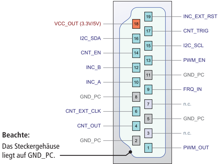
Abb. 23: HDMI-Steckverbinder (STB18)
