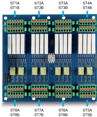
Abb. 4: Relaisboard ADQ-SCU-RB-16/8
