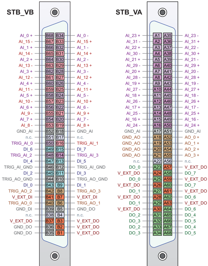
Abb. 27: Anschlussbelegung STB_VA und STB_VB
