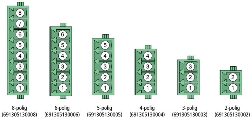
Abb. 9: Würth-Grundleiste (Draufsicht)
