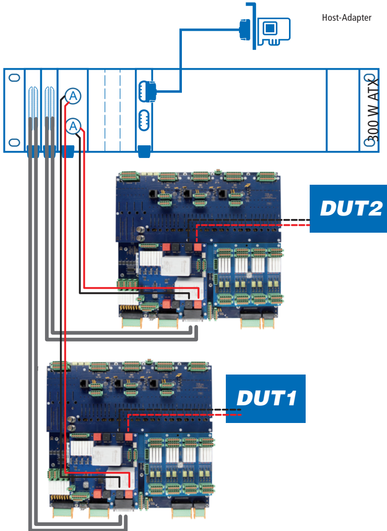
Abb. 7: Beispiel-Systemkonfiguration
