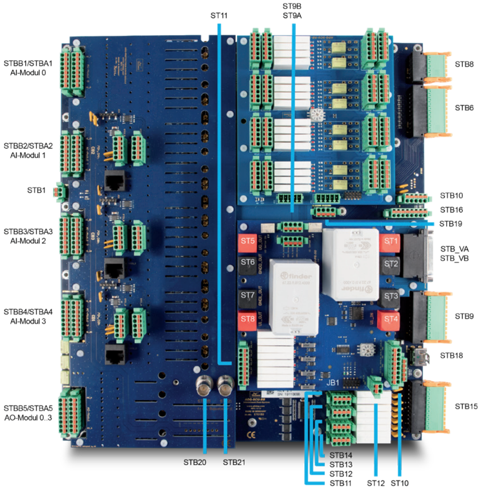
Abb. 8: Steckerpositionierung
