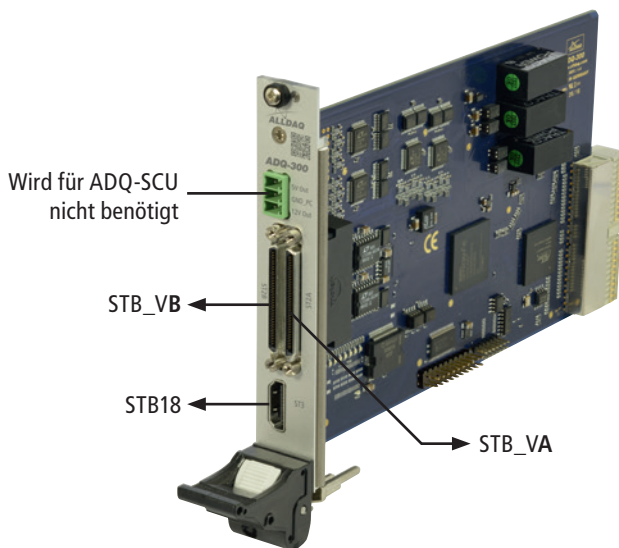
Abb. 6: Multifunktionskarte ADQ-348
