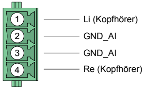
Abb. 24: Audio-Ausgang (STB19)
