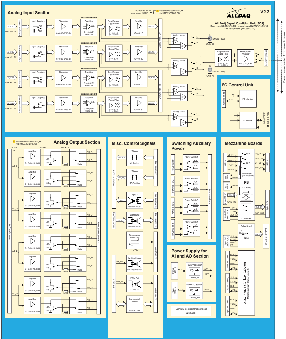
Abb. 1: Blockschaltbild ADQ-SCU
