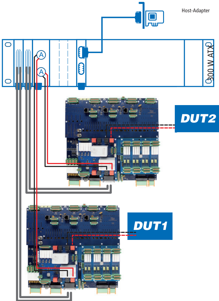
Abb. 7: Beispiel-Systemkonfiguration
