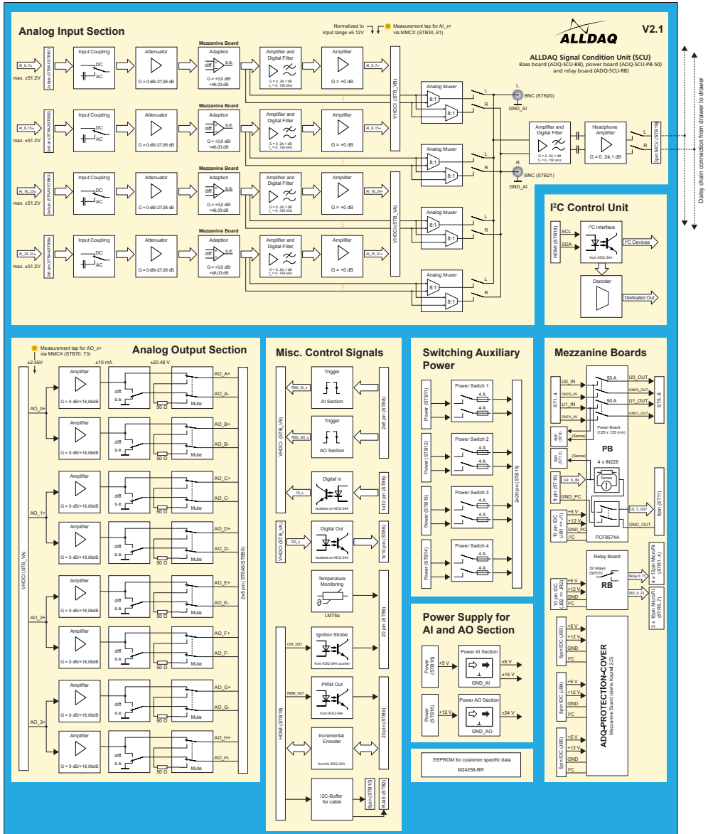
Abb. 1: Blockschaltbild ADQ-SCU
