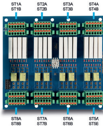
Abb. 4: Relaisboard ADQ-SCU-RB-16/8
